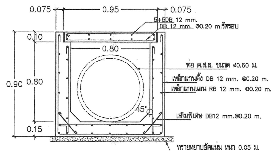
รูปตัด A-A
