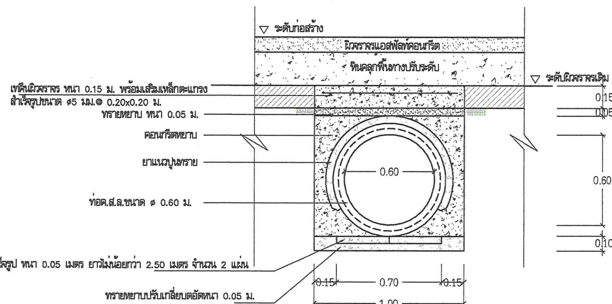
รูปตัดขยายท่อลอดถนน
