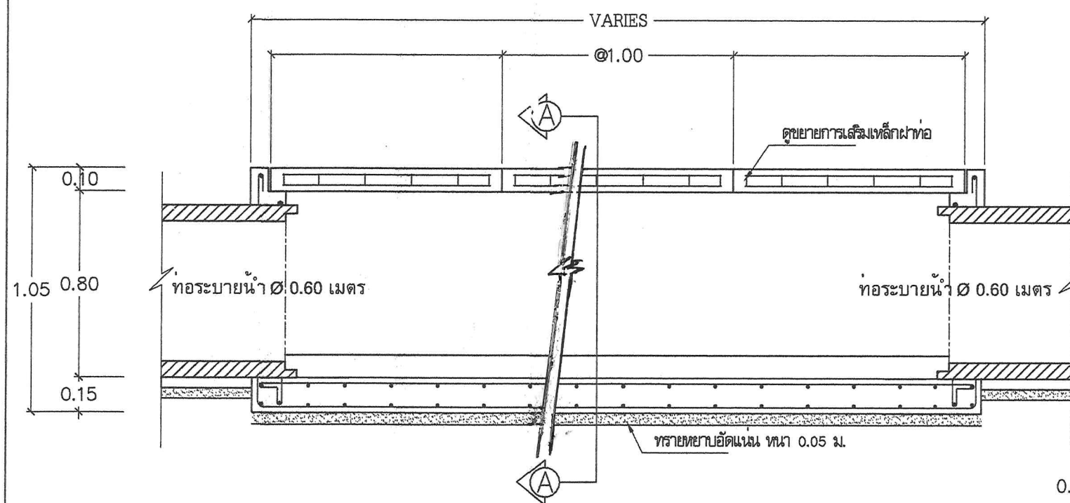
แบบการฝังท่อกรณีเกิดปัญหาอุปสรรค
