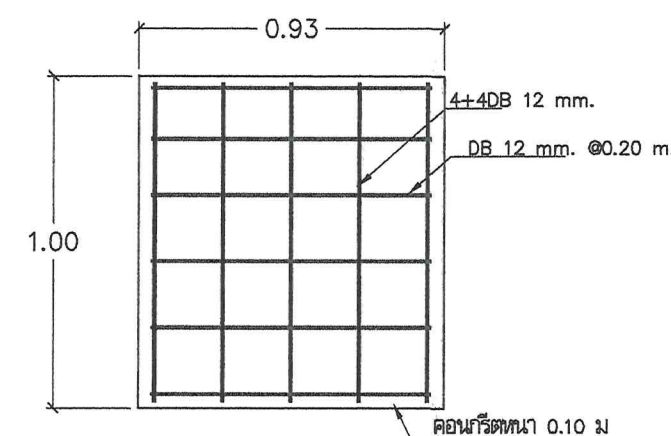
ขยายการเสริมเหล็กฝาท่อ
