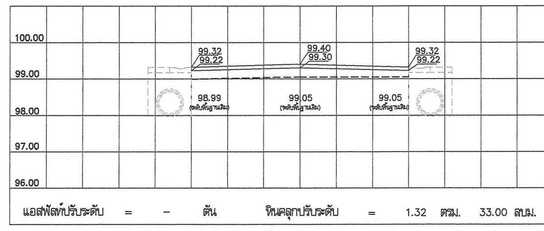
STA 0+650
