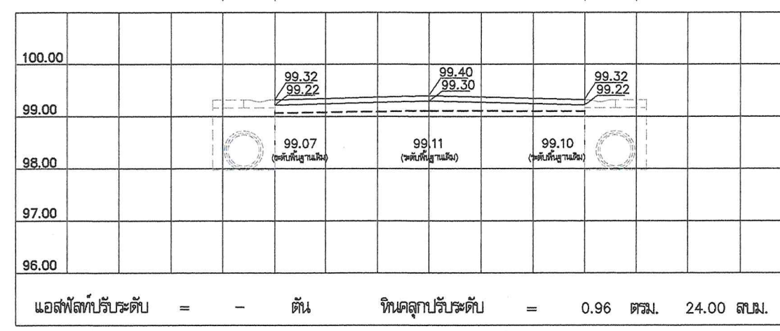
STA 0+625
