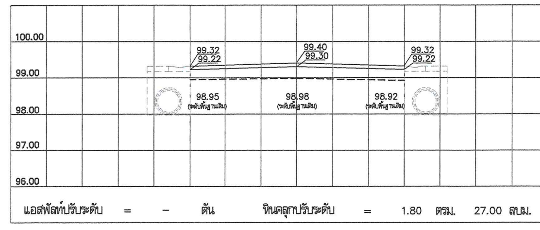
STA 0+675
