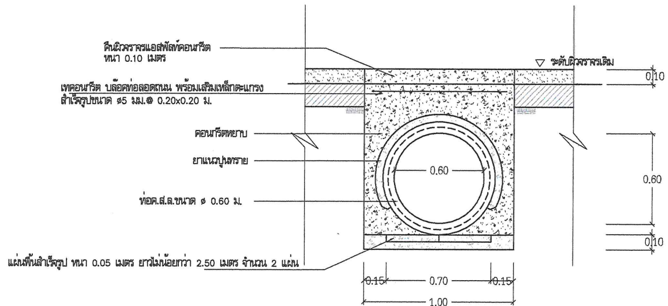
ขยายการฝังท่อลอดถนน
