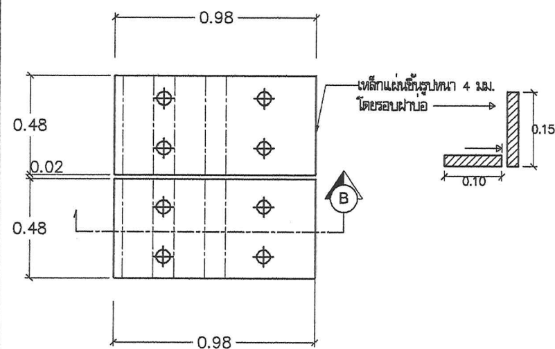
แปลนบ่อพัก
