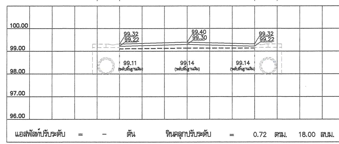
STA 0+600
