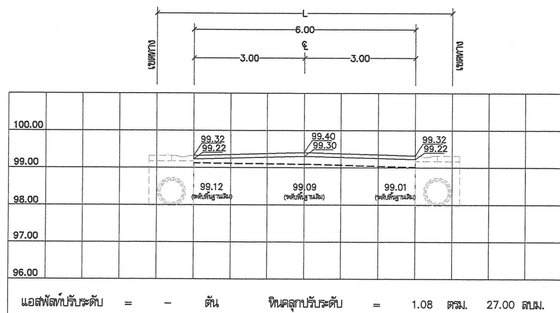
STA 0+250
