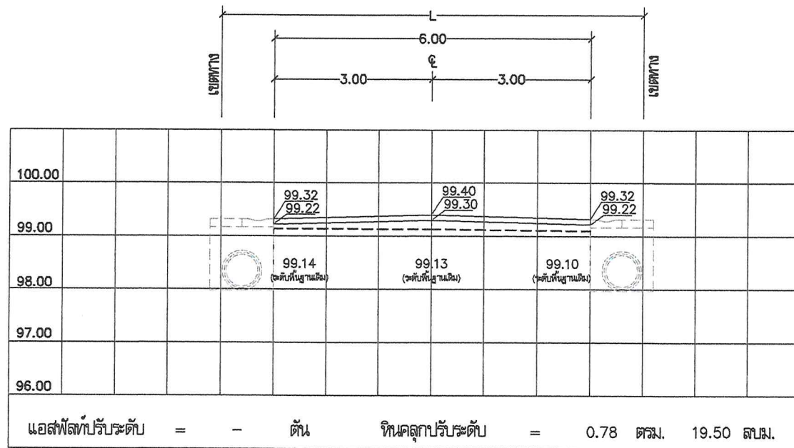
STA 0+200
