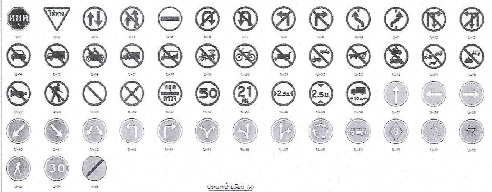
ประเภทป้ายบังคับ (บ)
