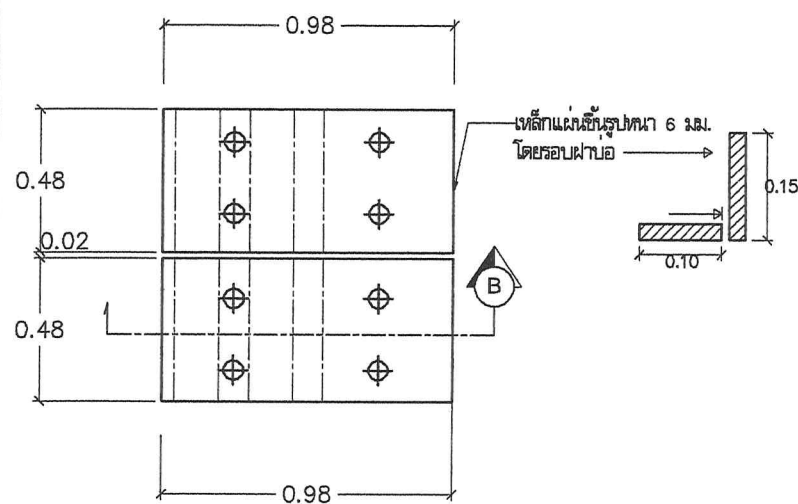
แปลนผ่าบ่อพัก
