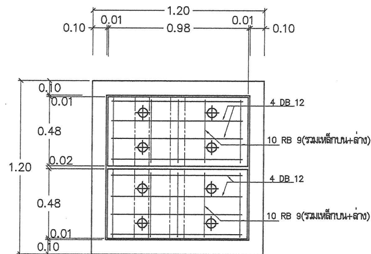
แปลนผ้าอปก(ขยายการเสริมเหล็ก)
